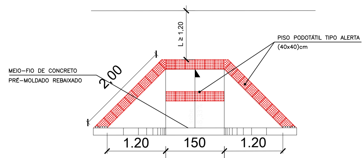
2 DETALHE RAMPAS DE ACESSO
